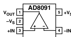
SOT23-5 (RT-5)
