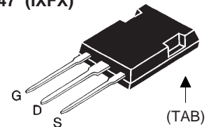
PLUS247 (IXFX)
