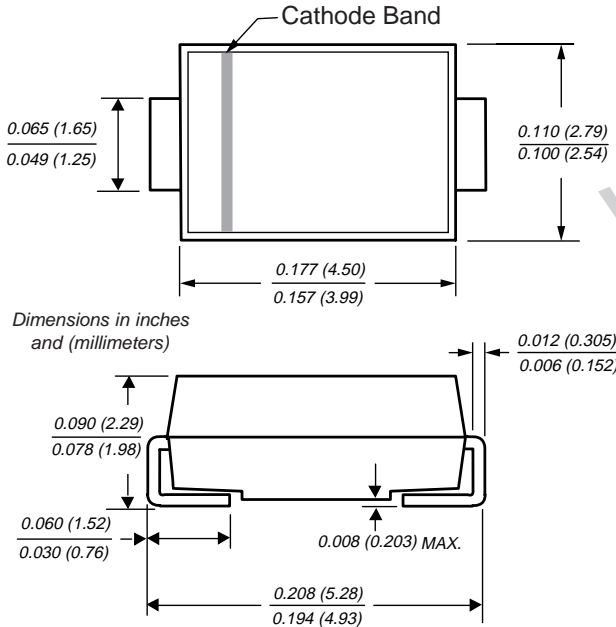
DO-214AC (SMA)
