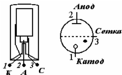
Рис. 1 Порядок расположения электродов тиратрона тлеющего разряда МТХ-90
