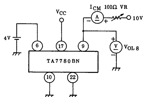
TEST CIRCUIT 8 : VOL9
