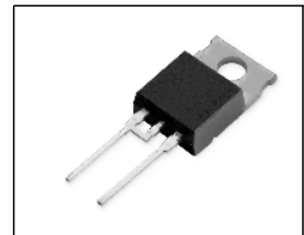
P-TO220-2-2.
