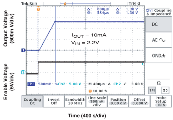
Enable Delay
