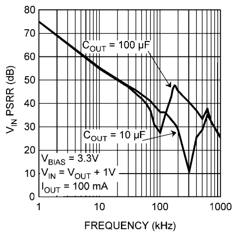
V_{IN} PSRR
