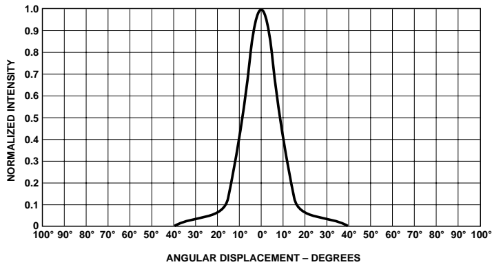
Figure 8. HLMP-Q106/-Q156.
